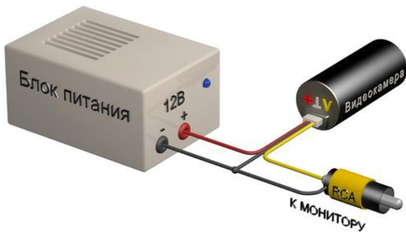
Схема подключения видеокамеры VB21HQX-W36
